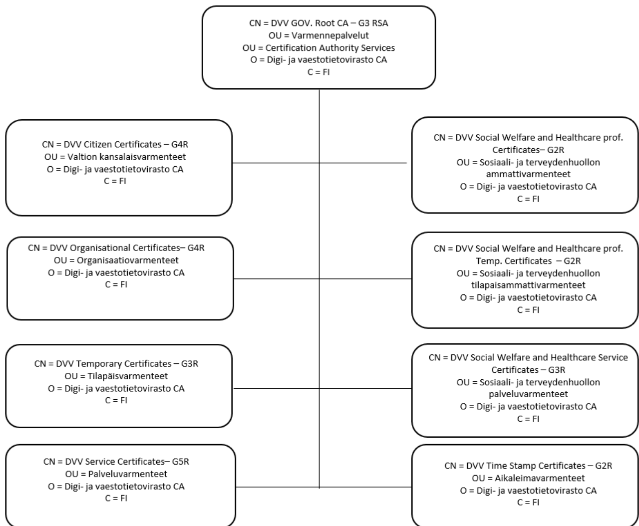
Bild 1: Certifikathierarkin RSA
