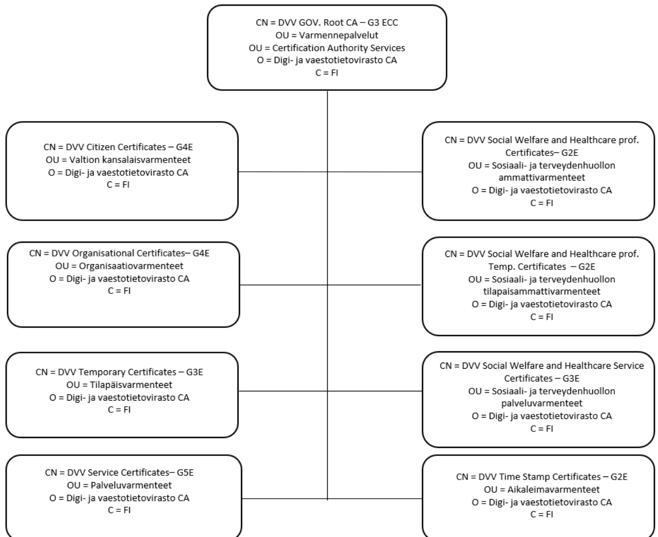
Bild 2: Certifikathierarkin ECC
