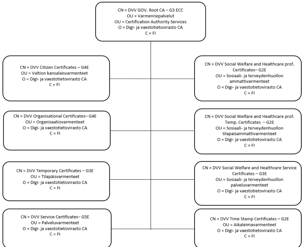
Kuva 2: Varmennehierarkia ECC
