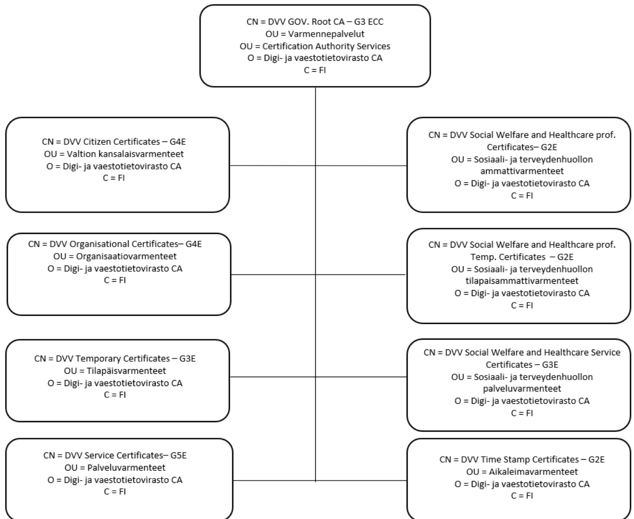
Bild 2: Certifikathierarkin ECC
