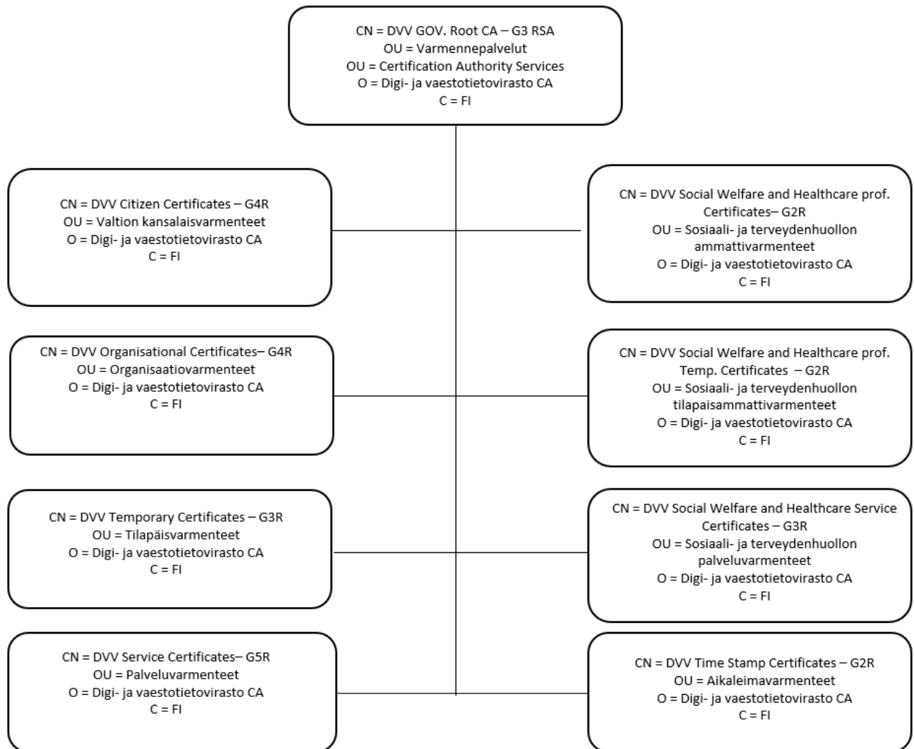
Bild 1: Certifikathierarkin RSA
