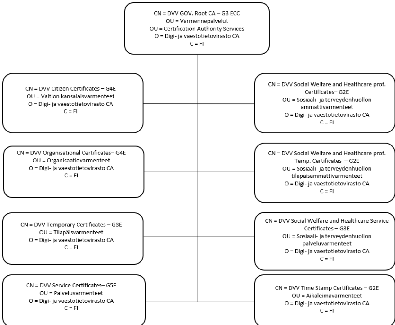
Bild 2. Certifikathierarkin ECC
