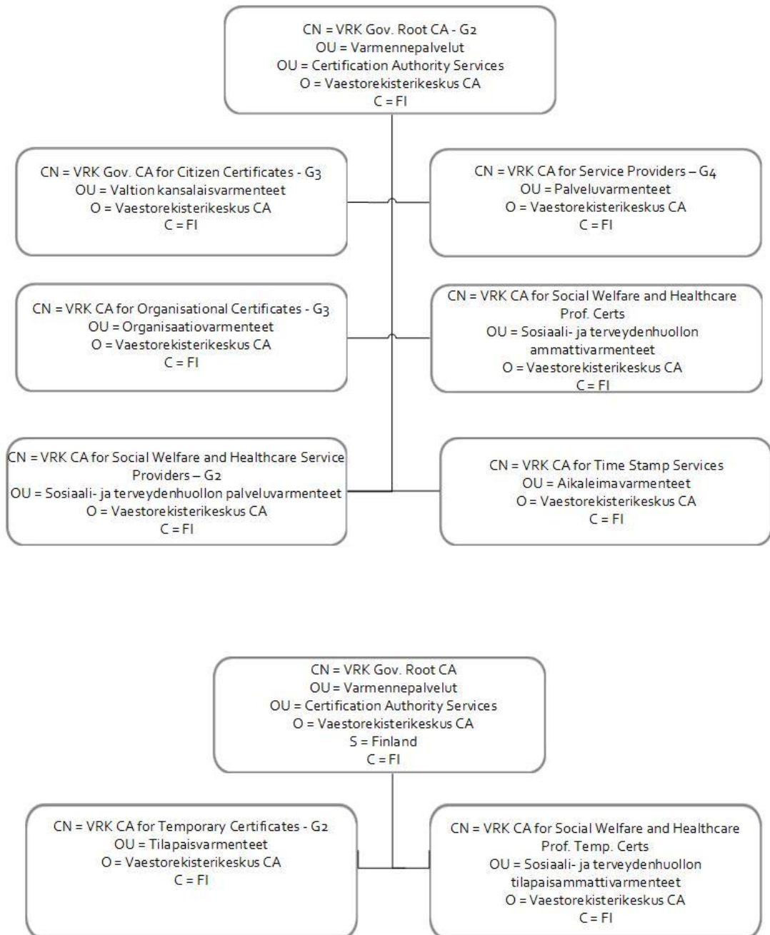
Kuva 1. Varmennehierkia.
